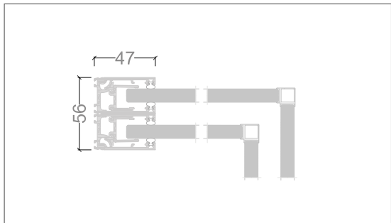
90° ANGLE
