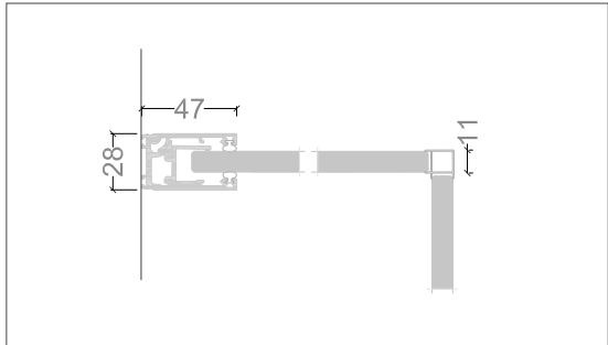
90° ANGLE
